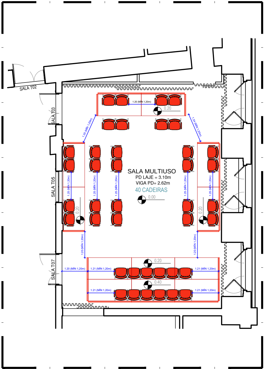
02 PLANTA BAIXA | SALA MULTIUSO | LAYOUT ARENA escala : 1/100
