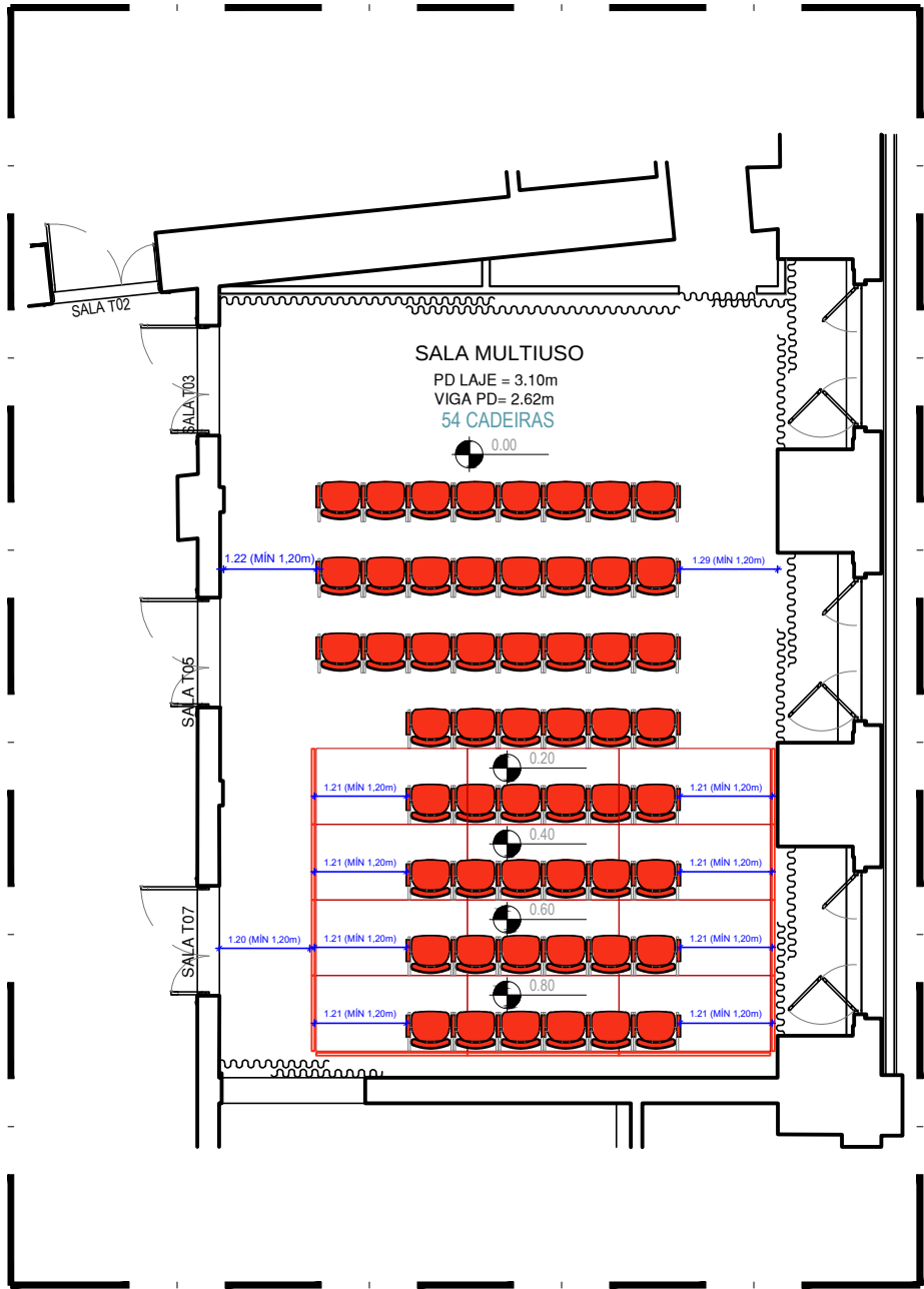
01 PLANTA BAIXA | SALA MULTIUSO | LAYOUT ITALIANO escala : 1/100
