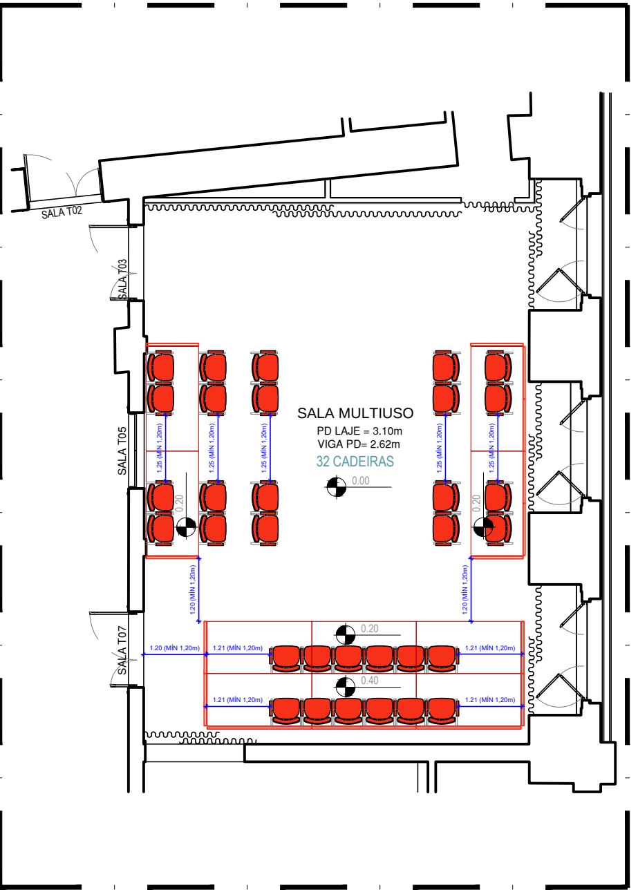
03 PLANTA BAIXA | SALA MULTIUSO | LAYOUT SEMI-ARENA escala : 1/100
