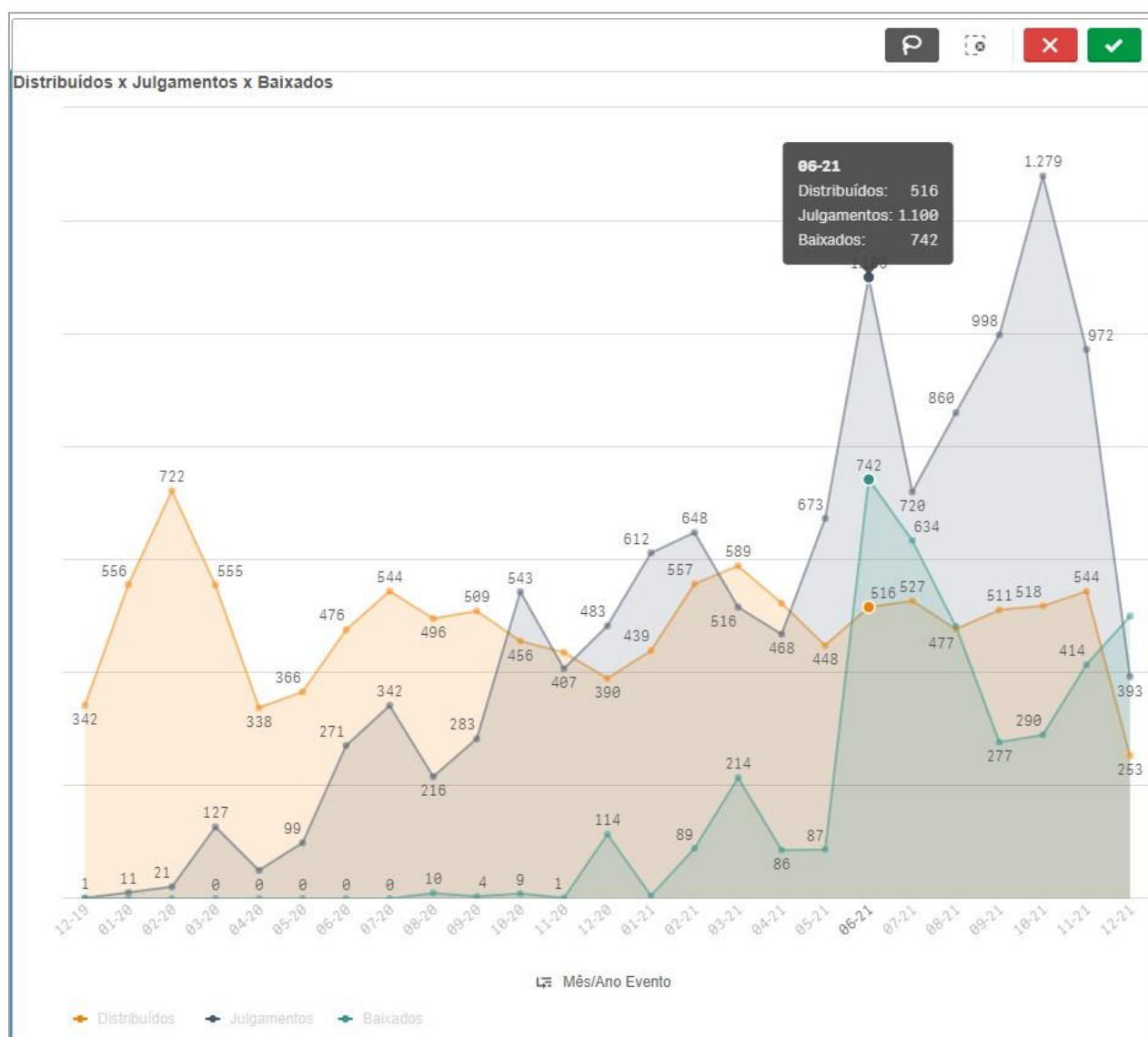
Figura 25– Detalhamentos dos Gráfico Movimentação
