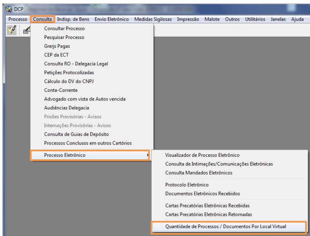
Figura 2 – Menu Consulta.
